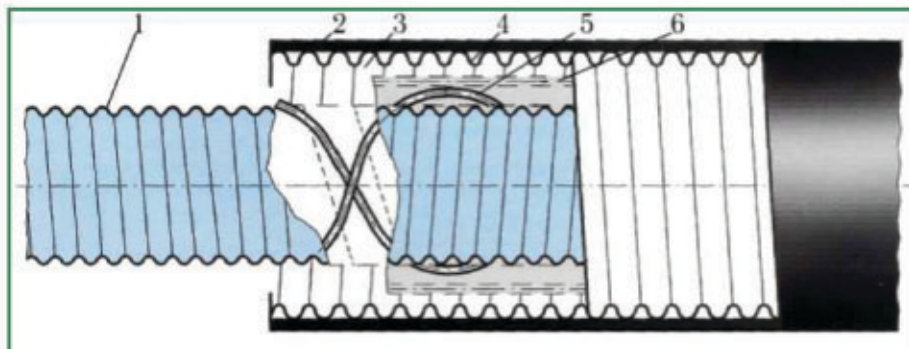
Рис. 4. Разрез криогенного трубопровода «Криофлекс»: 1, 4 — спиральные сварные трубопроводы (внутренний и внешний) из нержавеющей стали; 2 — защитная наружная цилиндрическая оболочка из полиэтилена; 3 — вакуумное пространство; 5 — спейсер; 6 — многослойная экранно-вакуумная теплоизоляция из полиэтилентерефталатной плёнки (ПЭТ) с двух сторон металлизированной алюминием
